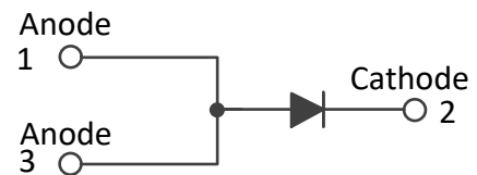
TO-263AB(D²PAK)
